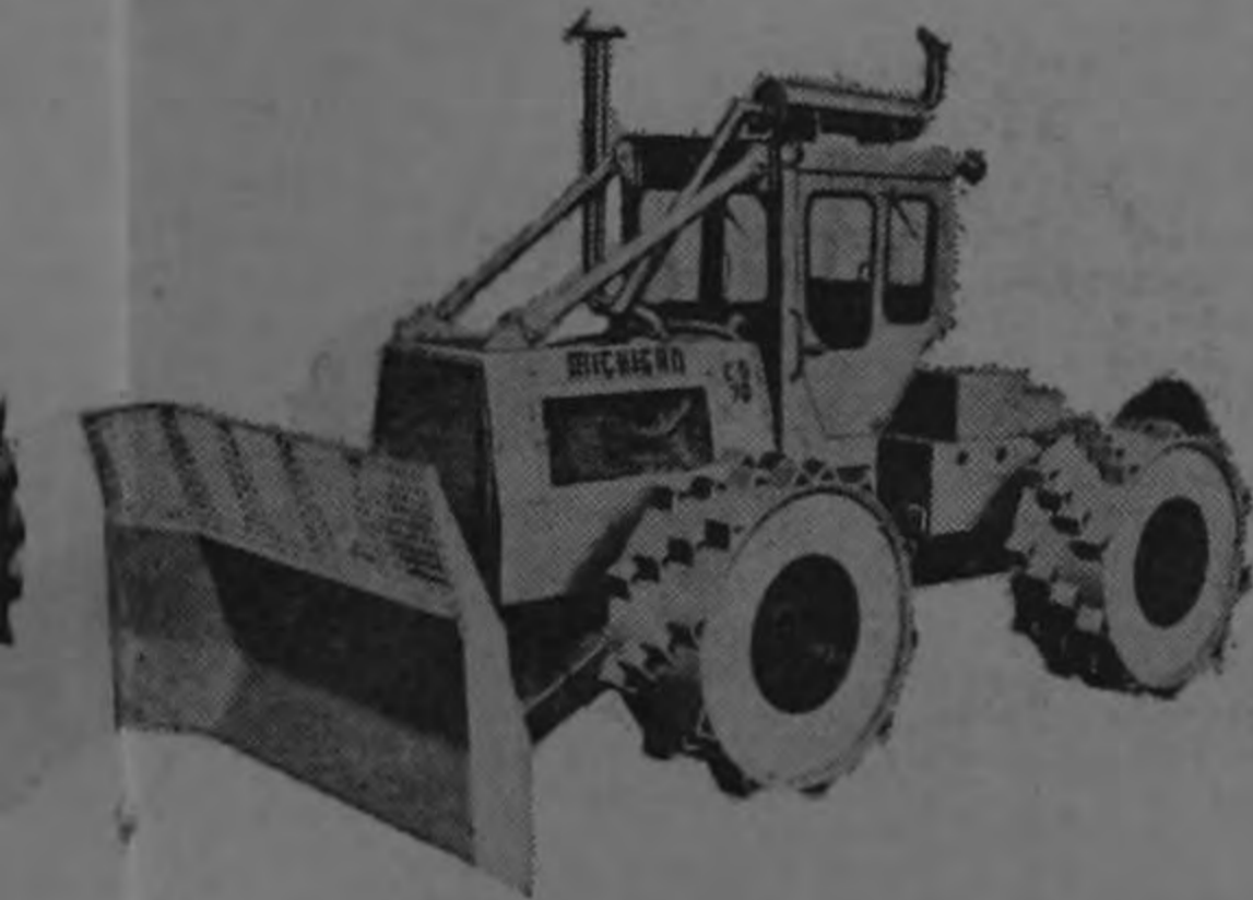
EQUIPOS ESPECIALES PARA LA COMPACTACION DE BASURA de 24.000 libras.
